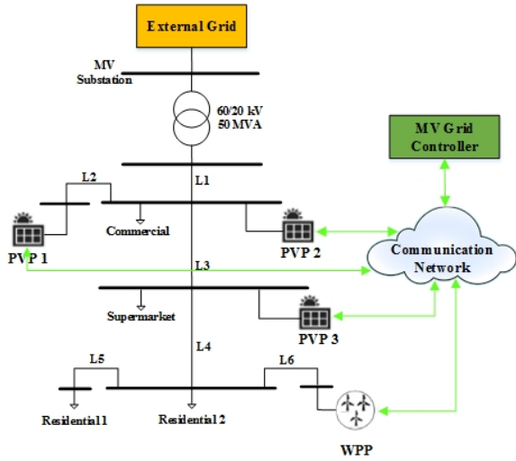
Fig. 1: Microgrid Scenario
